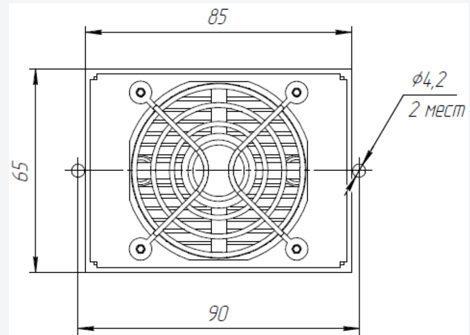
Схема монтажа
